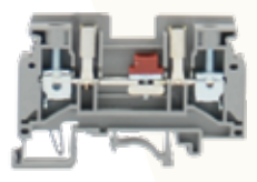
DCTK6N Kovansız
