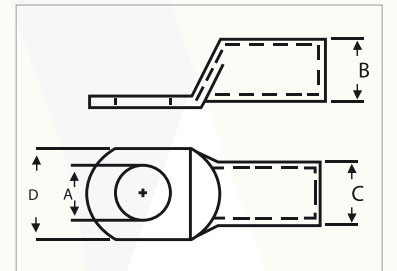
MKP - S
