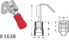
MPB 1638
